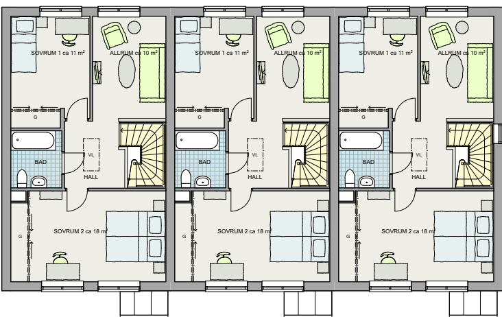
Planlösning tillval med två sovrum och allrum ▼
